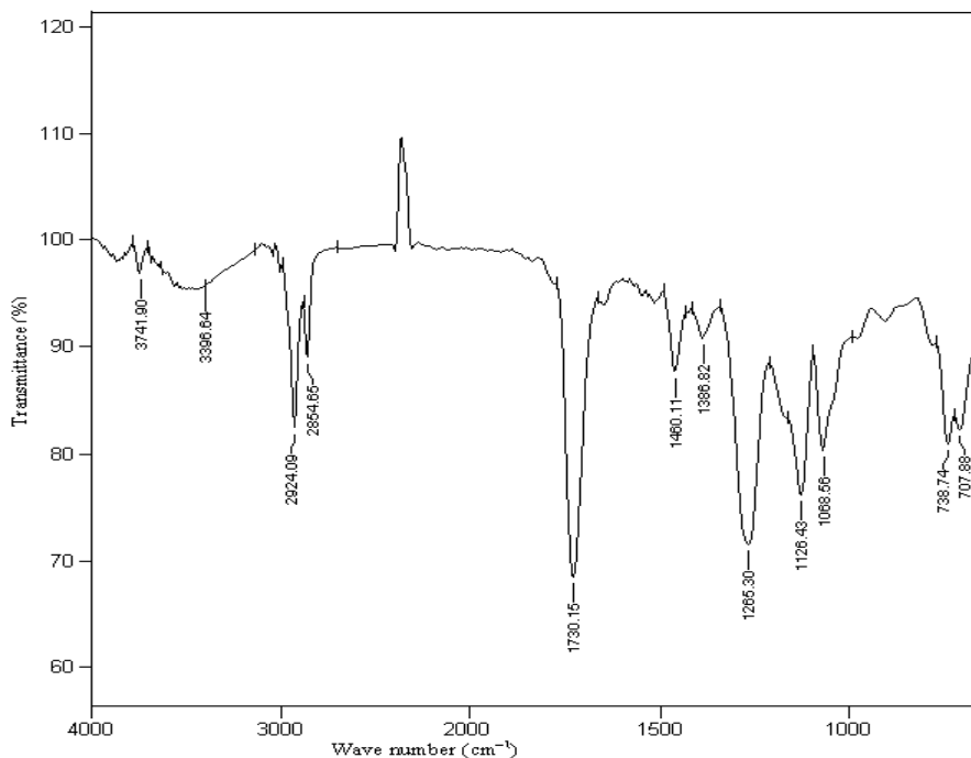
Figure3. FTIR spectra of pentaerythritol phthalic anhydride Resin
